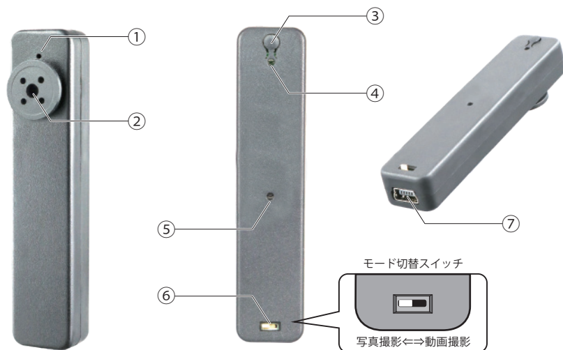
①マイク ②レンズ ③電源/撮影ボタン ④ステータスランプ[青][黄] ⑤リセットボタン穴 ⑥モード切替スイッチ ⑦USB接続口
