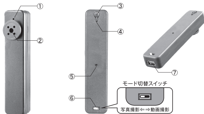
①マイク ②レンズ ③電源/撮影ボタン ④ステータスランプ ⑤リセットボタン穴 ⑥モード切替スイッチ ⑦USB接続口
