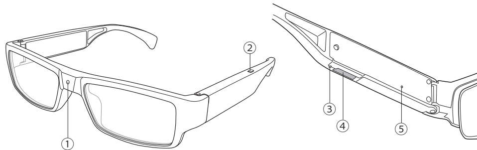
① カメラレンズ ② 電源／撮影ボタン ③ リセットボタン穴 ④ USB接続口 ⑤ ステータスランプ
