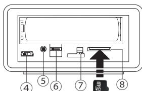
【製品裏面】※裏蓋を外した状態
